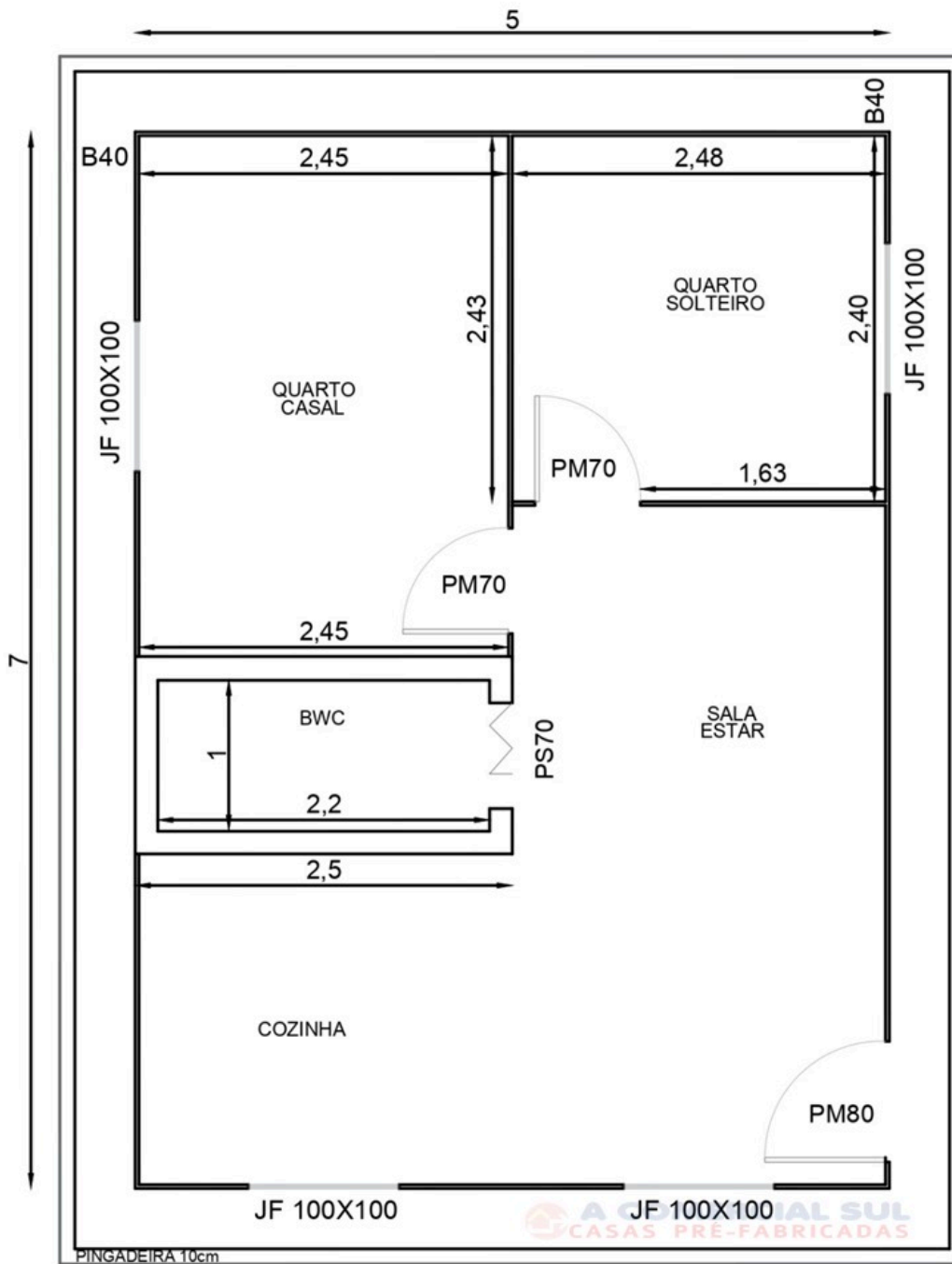
CASA 35m 2 35m 2 - 5,00 X 7,00
