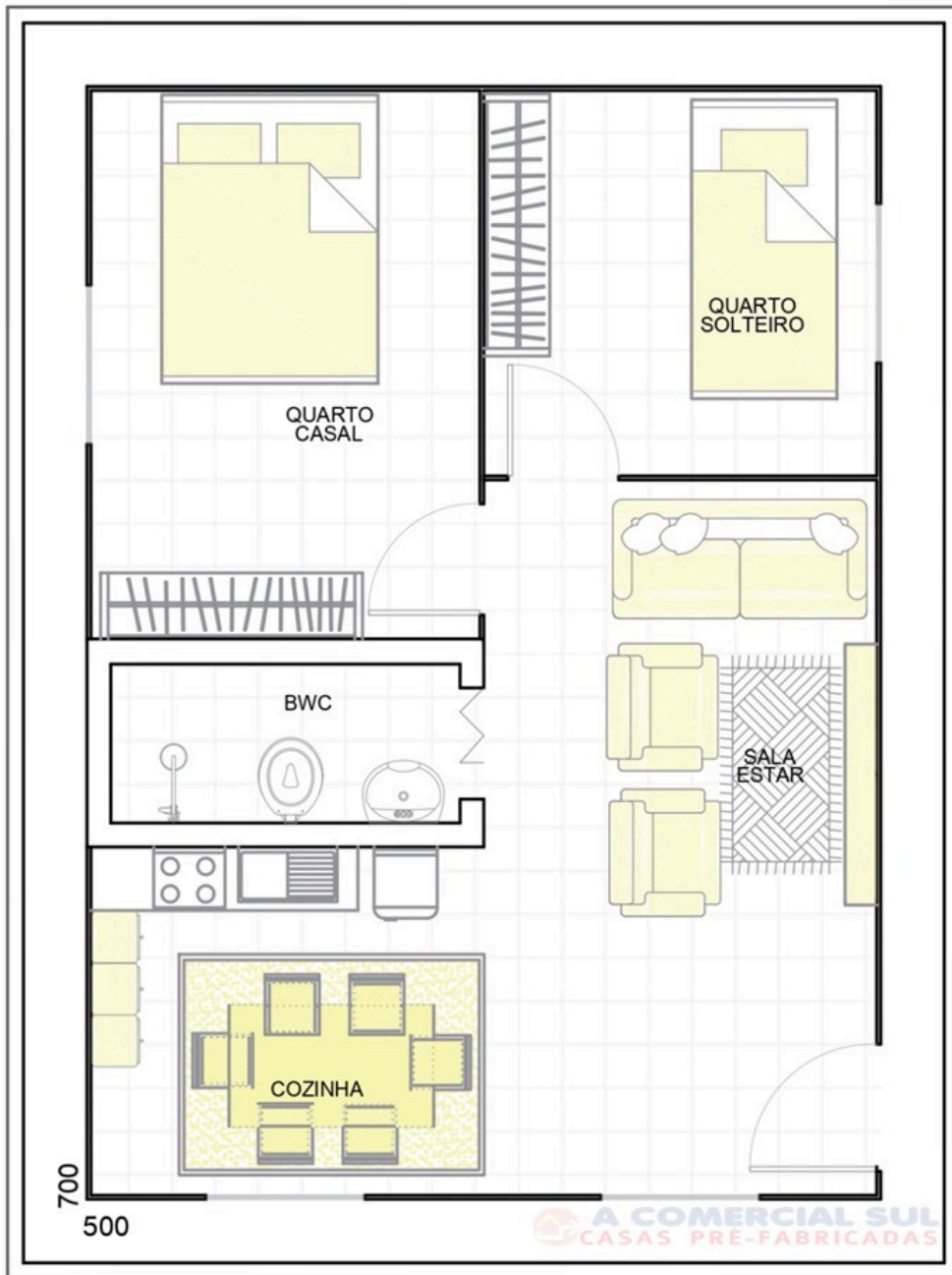
CASA 35m 2 35m 2 - 5,00 X 7,00
